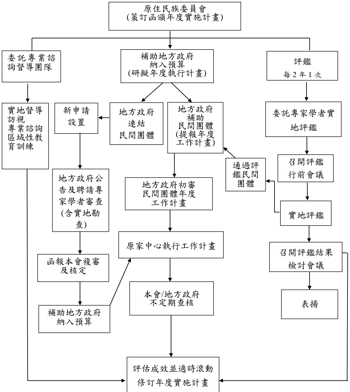
圖 2：運作架構圖
